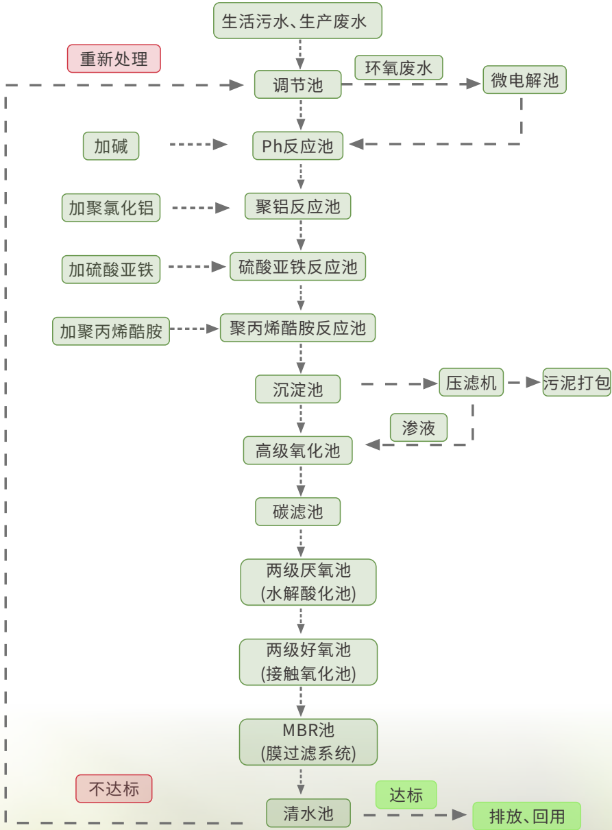
污水处理工艺流程图
